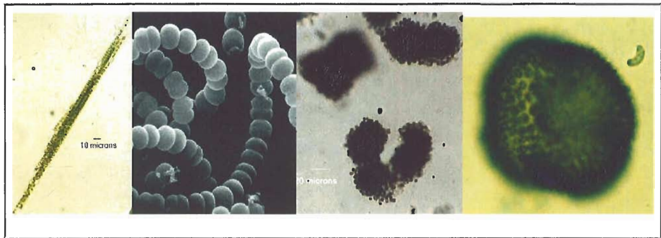
Aphanizomenon
