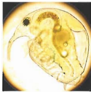
Bosmina longirostris
